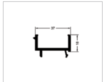
Hareketli lameller için tutma profili
