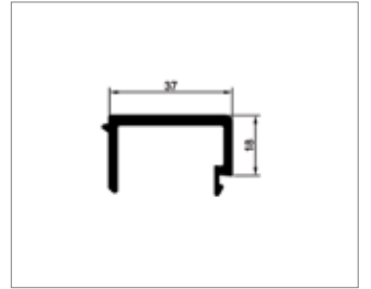
Delikli/deliksiz tutma profili
